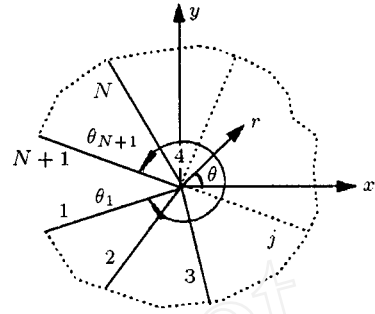
图 2 N 种材料切口示意图
