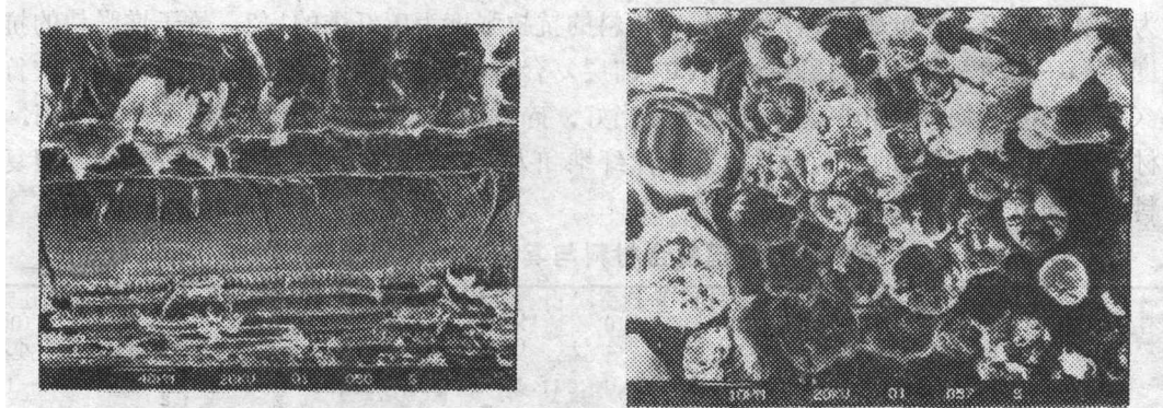
图3 竹薄壁细胞纵向
