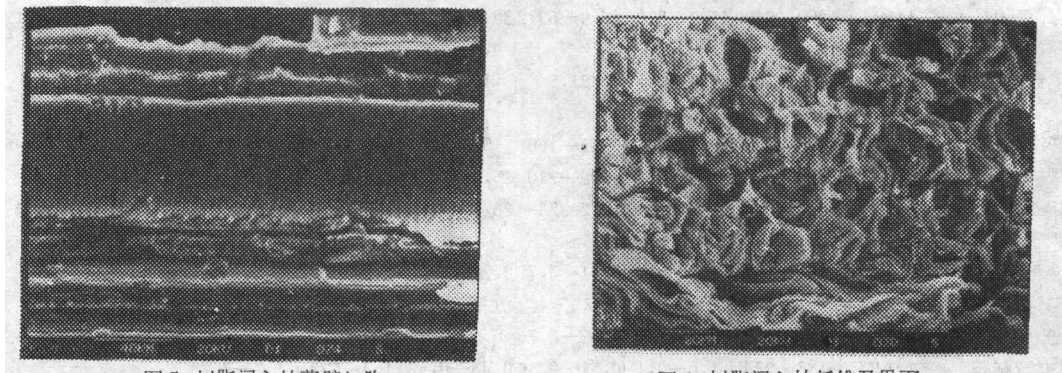
图5 树脂浸入竹薄壁细胞
